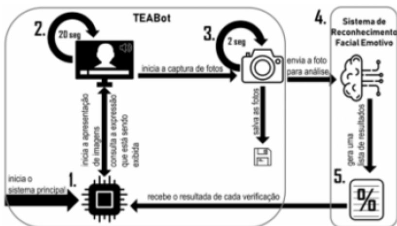
Figura 2: Arquitetura geral do sistema do robô TEABot
